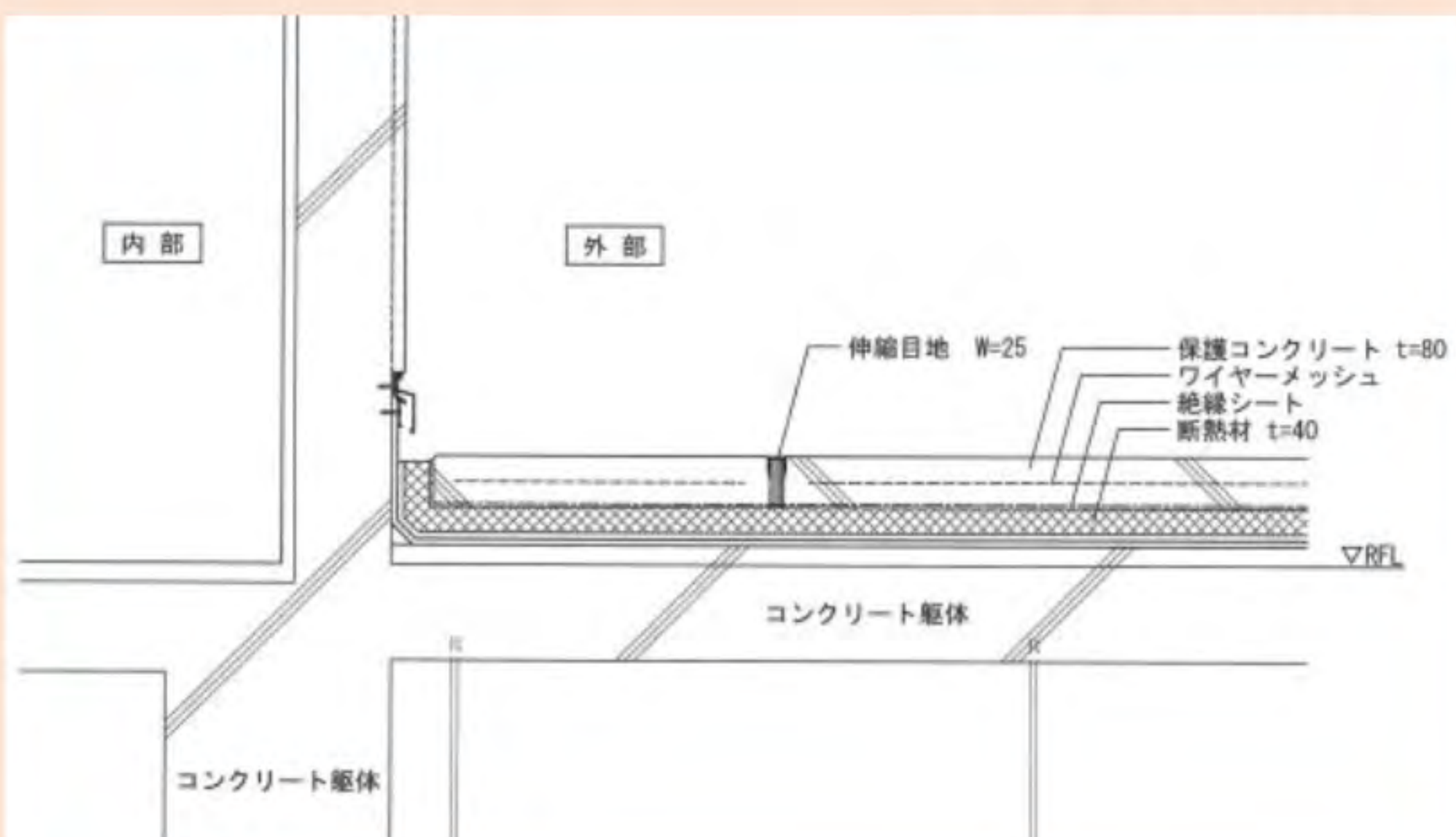
⑧断熱材の施工 アスファルトにて断熱材（厚さ4センチ）を張り付けます。
