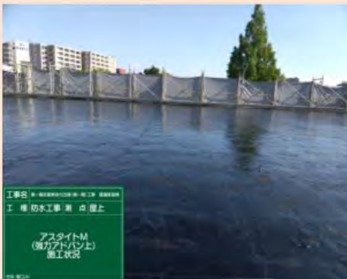
⑦アスファルト塗布 アスファルトを規定量塗布します。
