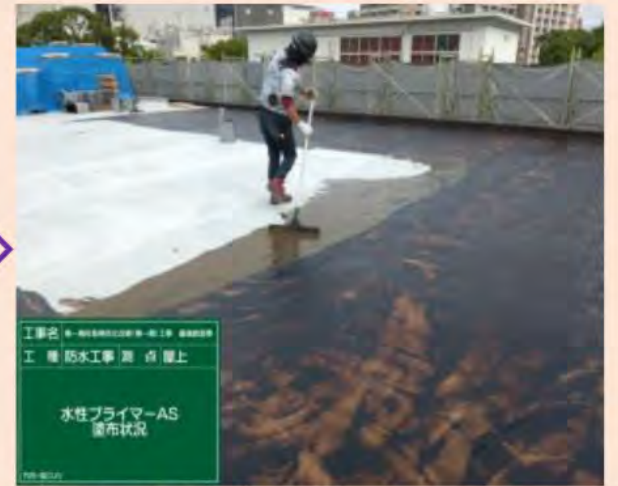
③プライマー塗布 清掃確認後、プライマーを均一に塗布します。
