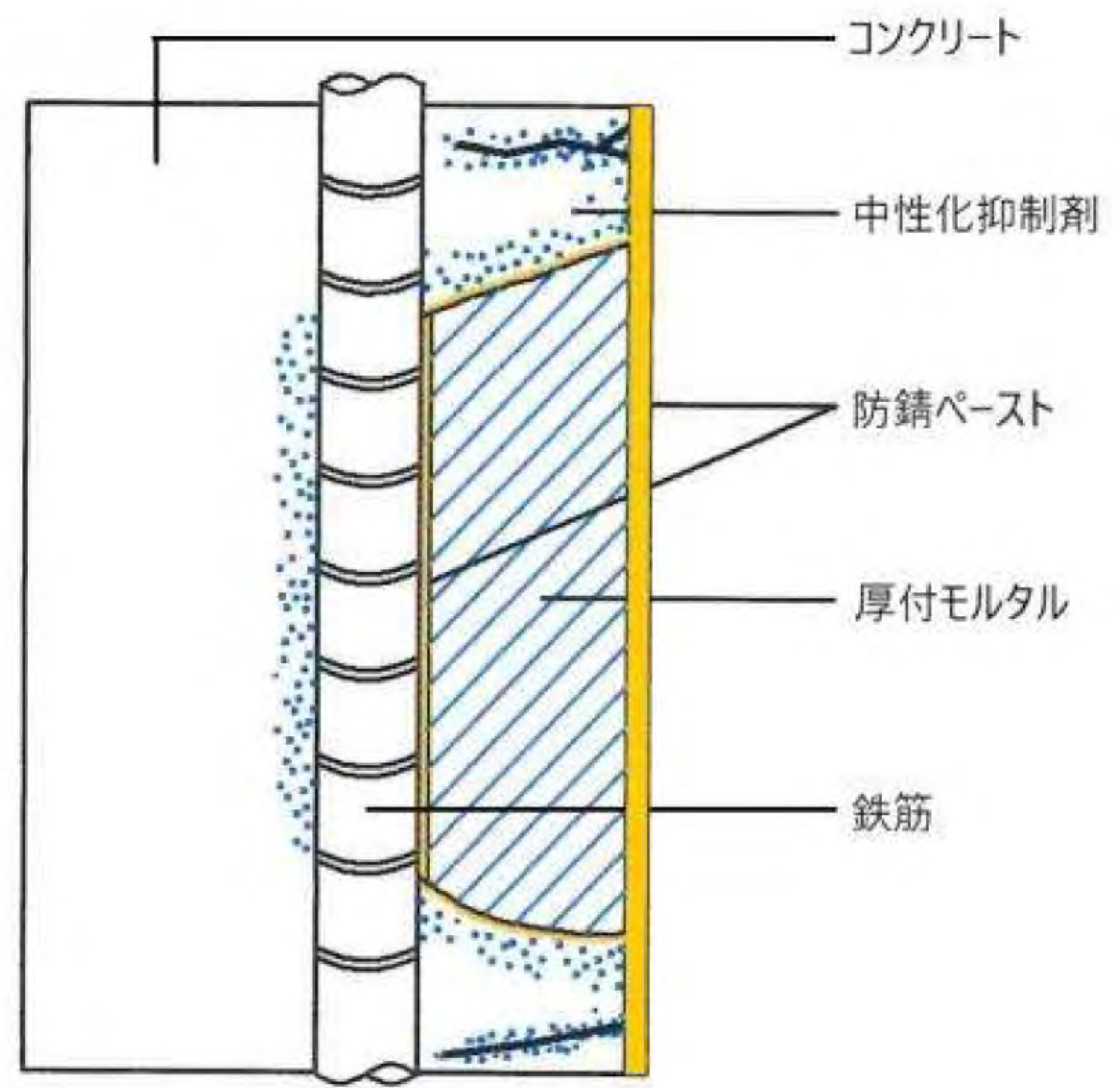
普通教室棟 壁模式図
